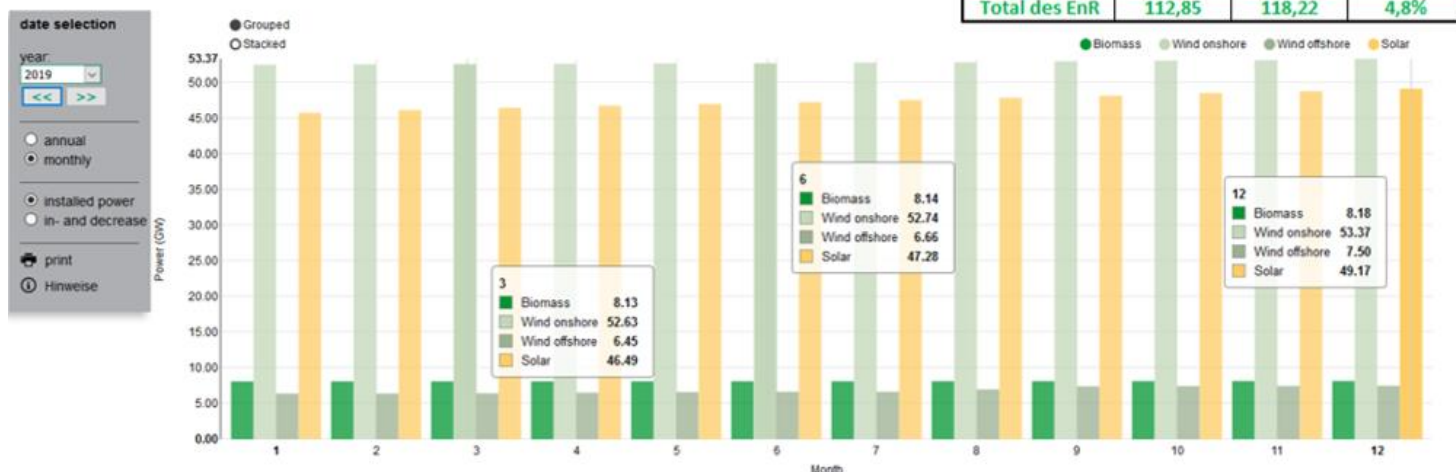
Évolution du parc renouvelable au long de l'année 2019 (src : Fraunhofer)
