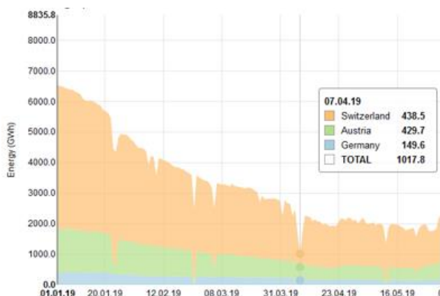
Évolution du stock hydraulique
