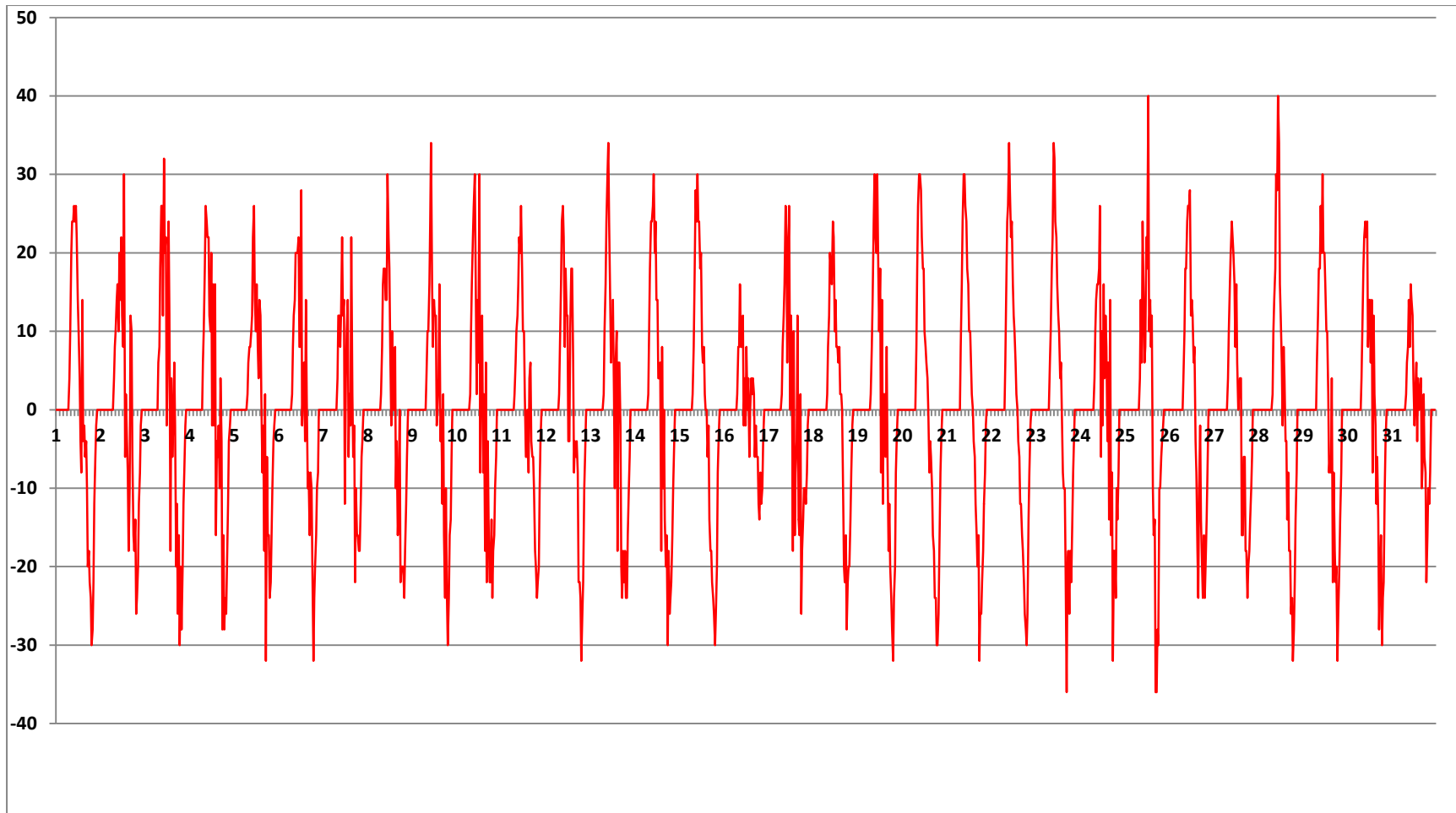
Fig.12 Gradient de puissance solaire (MW/h) Bretagne – Août 2013 Comme il se doit les gradients sont en moyenne directement liés au pic de production solaire. Ils sont positifs le matin et négatifs l'après-midi. Leur amplitude est aussi en relation avec la hauteur du pic. Plus il y a de soleil, plus le parc photovoltaïque exerce de contrainte sur le réseau. Ainsi pour des pics dépassant 100 MW en milieu de journée les gradients peuvent dépasser +/- 30MW/h. Surimposé à cette tendance générale, on observe aussi des irrégularités à l'échelle de la demi-heure qui, si elles ne correspondent pas une incertitude de la collecte de données par RTE/eCO2mix, pourraient être attribuées à l'effet « un nuage passe ».
