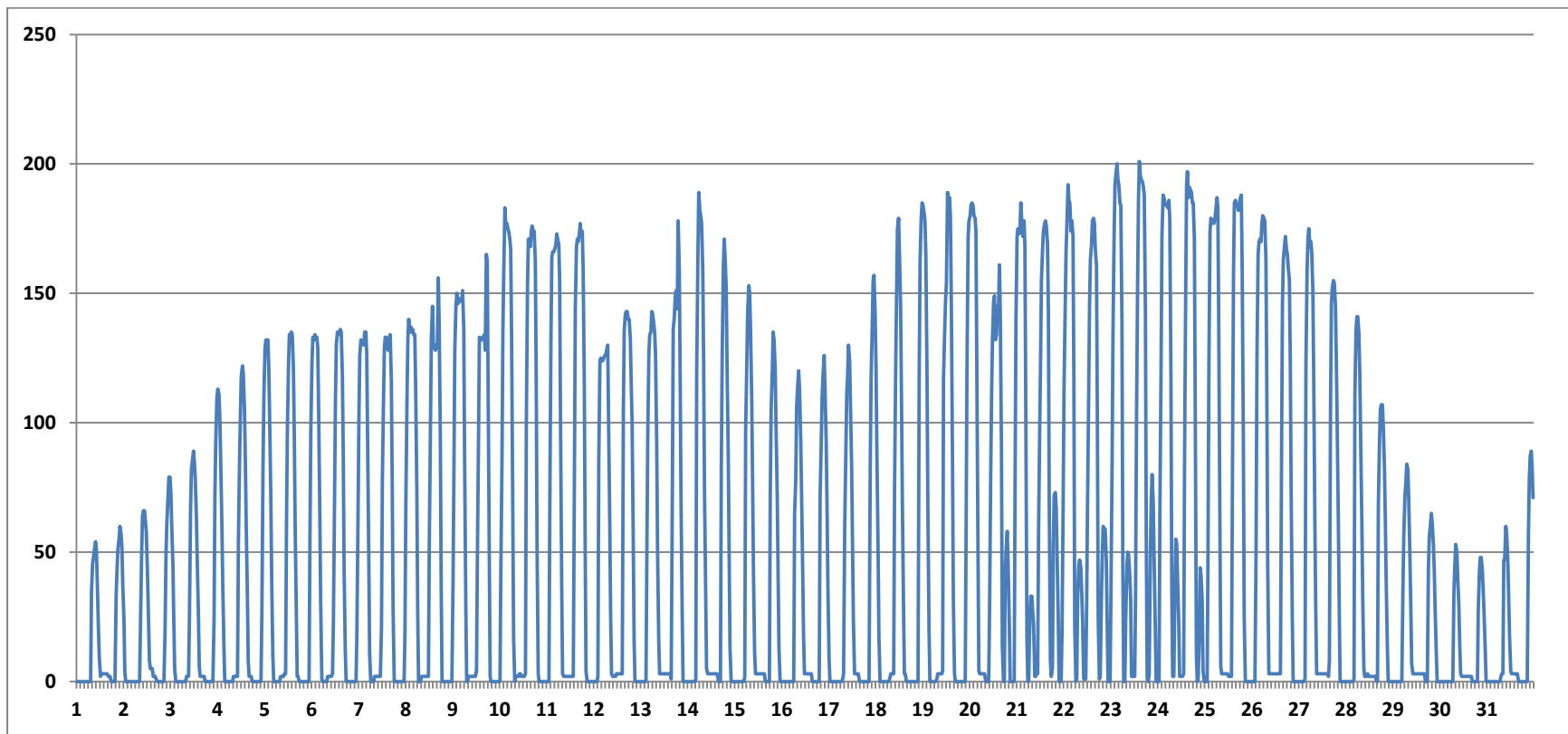
Fig.13 Production hydraulique, Puissance (MW) Bretagne – Août 2013. L'hydraulique breton lié au barrage de la Rance se distingue du reste de l'hydraulique français (de type « fil de l'eau » ou « éclusées »). C'est non seulement une énergie fatale (comme l'hydraulique de fil de l'eau) mais aussi une production au rythme alternatif. Elle ne participe que faiblement au réglage du réseau par le biais d'une fonction de pompage. L'énergie totale livrée au réseau sur le mois a été de 39,4 GWh (mois précédent 34,3 GWh), alors que le pompage (une consommation de courant restituée pour partie ultérieurement et comptabilisée dans le total « hydraulique ») n'a concerné que 4,7 GWh. Difficilement visible sur cette figure, on peut vérifier un décalage horaire progressif des pics reflétant celui des marées (idem pour les pics de pompage non illustrés dans ce document). Les structures de production à « pic double » observable en seconde partie du mois, correspondent ce mois-ci à des périodes où il y a peu ou pas de stockage par pompage.
