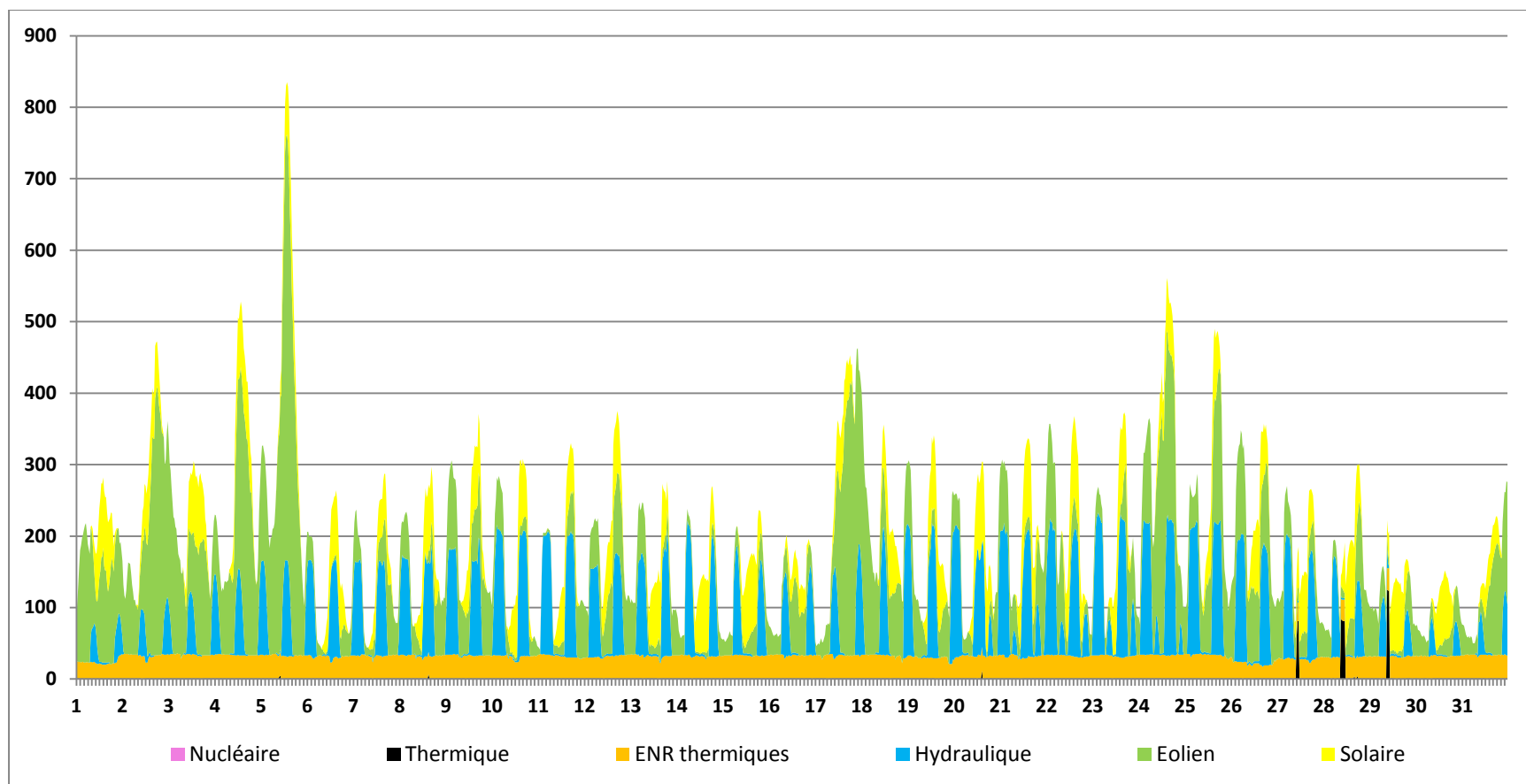
Fig.2 Production électrique de la Bretagne Août 2013 (MW). Ce mois-ci, l'ensemble de ces productions compte environ 11 % de la consommation locale. En GWh la production totale a été de 60,2 (mois précédent 87,3) pour l'éolien, 39,4 (mois précédent 34,3) pour l'hydraulique, 22,8 (mois précédent 20) pour les ENR thermiques et de 22,6 (mois précédent 23) pour le solaire (consommation totale 1434,7 GWh – mois précédent 1515 GWh). A l'exception des ENR Thermiques dont la production est quasi-constante et de la faible contribution thermique (1,2 GWh – mois précédent 1,5 GWh), les autres énergies, toutes fatales, fluctuent sans corrélation avec les besoins en électricité de la région. Comme l'attrait financier de subventions spécifiques accordées à la cogénération ne concerne que la période hivernale (Novembre à Mars), à l'exception de quelques pics, le thermique est arrêté ce mois. Tout comme l'ENR thermique qui fonctionne en base il ne participe pas à la gestion de régulation du réseau.
