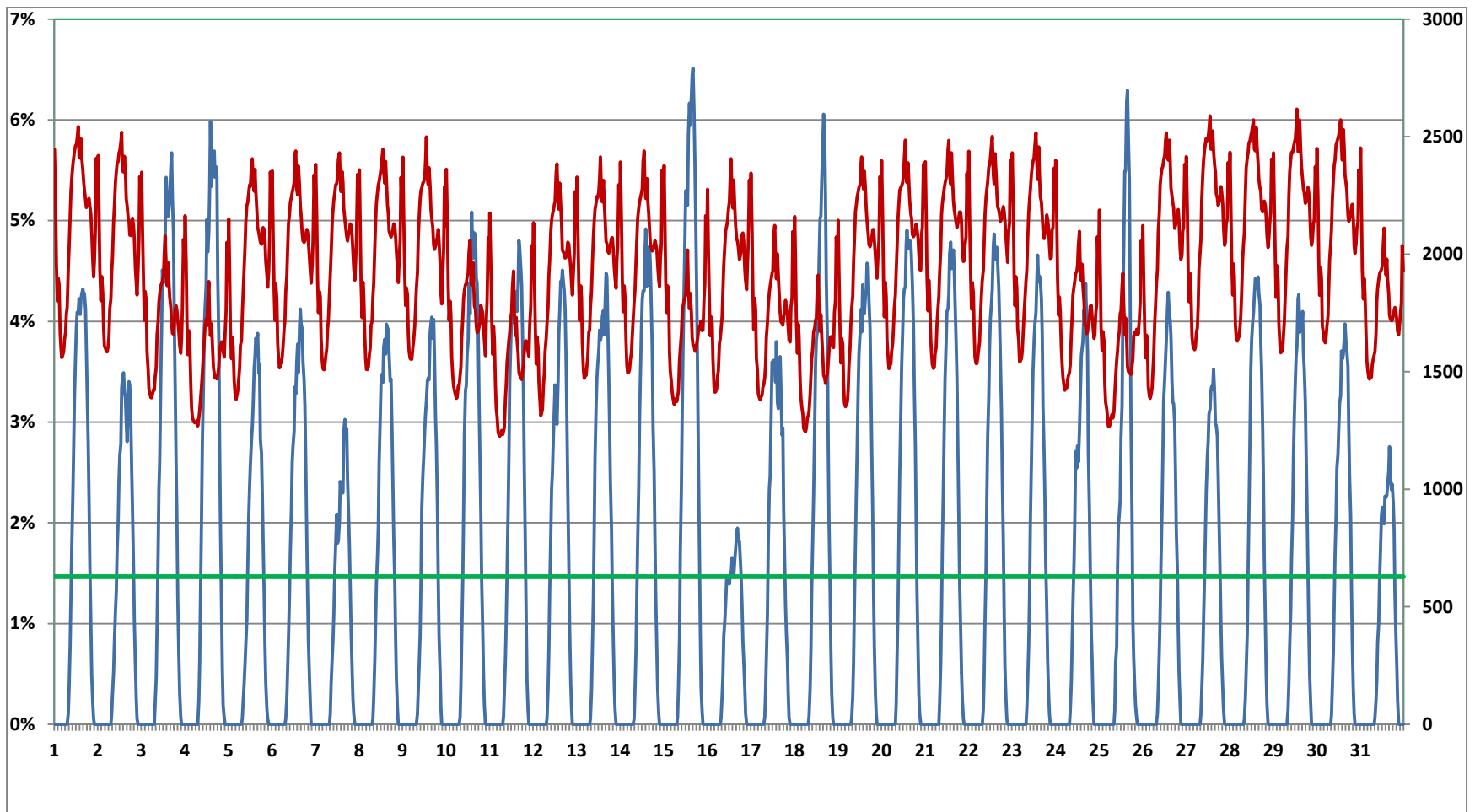
Fig.10 Production photovoltaïque, Taux de couverture (%) Bretagne – Août 2013. La courbe rouge (échelle de droite en MW) montre l'évolution de la consommation. En moyenne, le taux de couverture (rapport de la puissance livrée à la puissance consommée au même instant) du photovoltaïque est de 1,46 % (mois précédent 1,42 %). Il atteint son maximum de 6,5 % (mois précédent 6,3 %) le 15 du mois à 16h00 (fête de l'Assomption) quand le soleil est encore haut et que la consommation baisse. De façon générale, les meilleurs taux de couverture sont atteints les weekends à des moments où une bonne production photovoltaïque se combine à un faible besoin en électricité. Les pics du taux de couverture reflètent donc autant la production solaire que la faible consommation.
