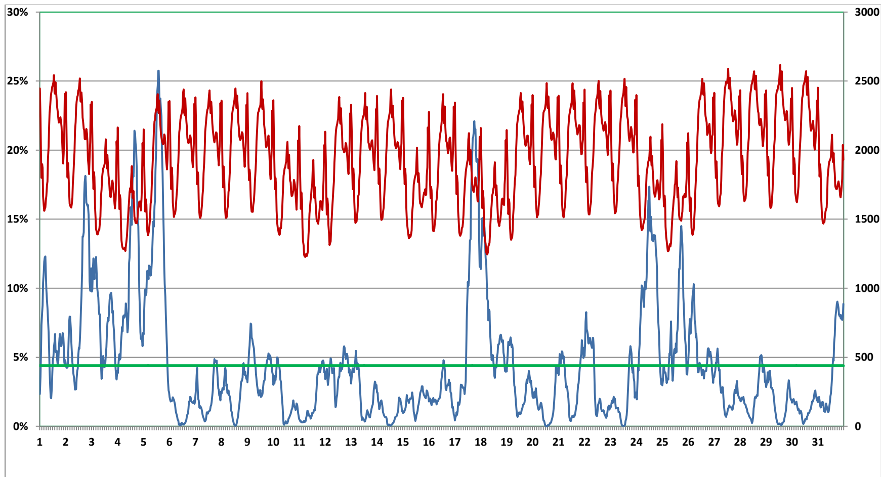
Fig.4 Production éolienne, Taux de couverture (%) Bretagne – Août 2013. La courbe rouge (échelle de droite en MW) montre l'évolution de la consommation. En moyenne, le taux de couverture (rapport de la puissance livrée à la puissance consommée au même instant) de l'éolien est de 4,4 % (mois précédent 6 %). Il atteint son maximum de 25,75 % (mois précédent 35,3 %) le 5 du mois à 14h00 (remarquablement, par rapport aux autres mois c'est un jour ouvré de cette période estivale). A cette exception près, les pics du taux de couverture reflètent autant la production éolienne que la faible consommation. Le minimum est de 0 % le 20 du mois à 12h00 (un jour ouvré).
