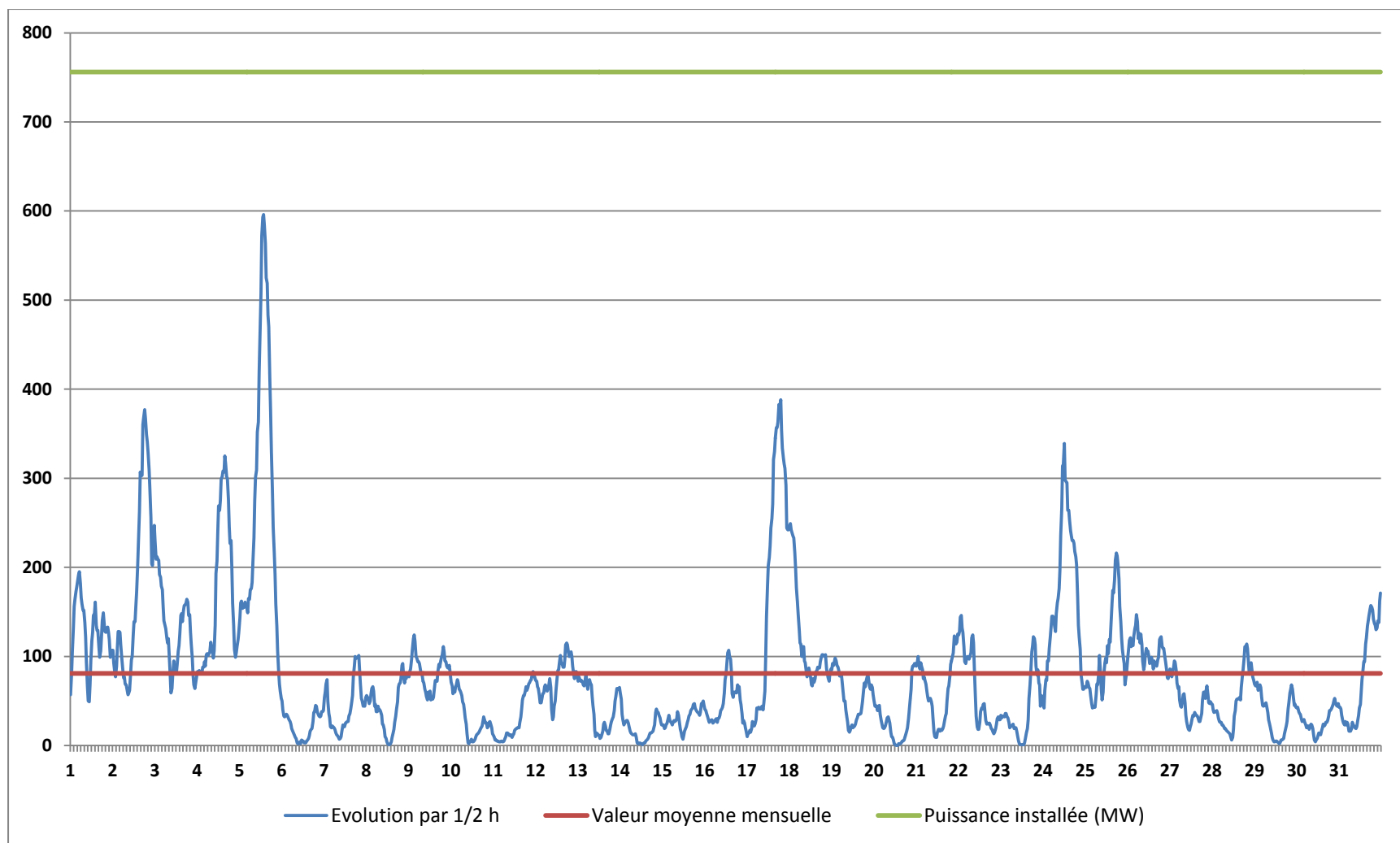
Fig.3 Production éolienne, Puissance (MW) Bretagne – Août 2013. En nous basant sur les données des 30/06/2013 et 30/09/2013 des « Tableaux de bord éolien et photovoltaïque » du ministère nous avons estimé la puissance éolienne régionale installée à 756 MW. La puissance moyenne livrée au réseau sur le mois a été de 81 MW (mois précédent 117,3) soit une efficacité moyenne de 10,7 % (mois précédent 15,5 %). Le maximum de production a été de 596 MW (mois précédent 521 MW) pour une efficacité 78,8 % (mois précédent 68,9 %) le 5 du mois à 13h30. Plusieurs fois dans le mois, la production a été quasi-nulle. Elle a été nulle le 20 du mois à 12h30.
