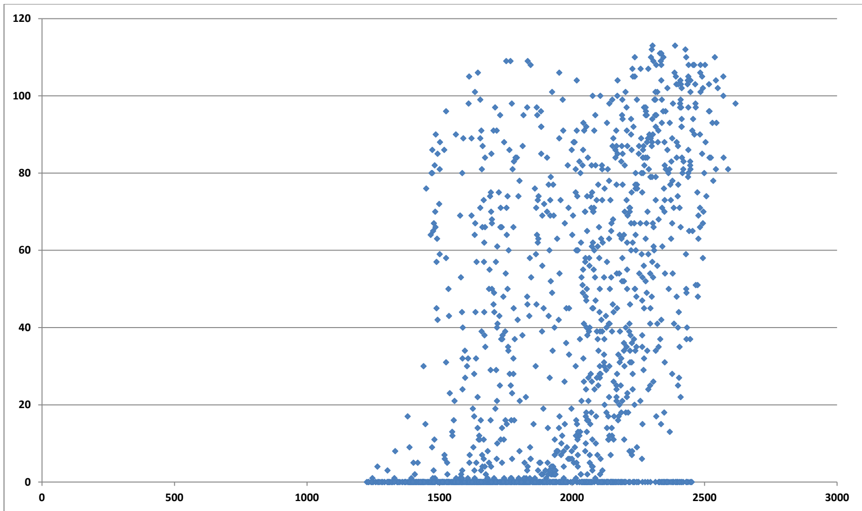
Fig.11 Bretagne Août 2013. Diagramme de corrélation entre la puissance photovoltaïque livrée (axe vertical unité MW) et la consommation au même instant (axe horizontal MW). Alors que la consommation électrique de la région est parmi les plus faibles de l'année, on observe encore ce mois-ci une corrélation plutôt positive (nuage de points incliné vers la droite sur la droite du diagramme). C'est donc quand il n'y a pas de véritable besoin que le solaire photovoltaïque semble montrer une certaine utilité.
