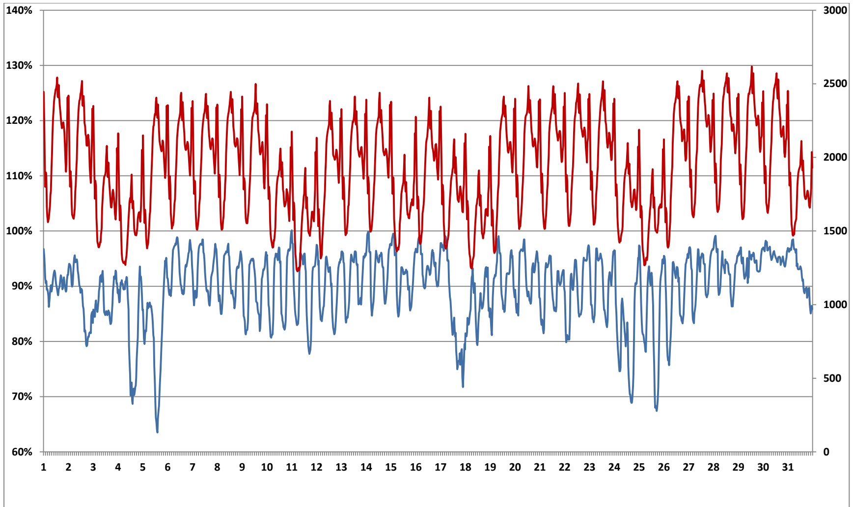
Fig.16 Importation électrique, Taux de couverture (%) Bretagne – Août 2013. La courbe rouge (échelle de droite en MW) montre l'évolution de la consommation. En moyenne sur le mois, le taux de couverture (rapport de cette puissance importée à la puissance consommée par la région au même instant) est de 89,9 % (mois précédent 89 %). A son maximum il atteint 100,1 % (mois précédent 101 %) le 11 du mois à 0h00. On a donc la démonstration que le barrage de la Rance sert à stocker de l'énergie – statistiquement d'origine nucléaire – qui devient de l'énergie « verte » lors du lâcher de l'eau. Au minimum, le taux de couverture d'importation est de 63,5 % (mois précédent 49,3 %). Il a lieu le 5 du mois à 14h00 au moment où en ce jour de weekend quand le taux de couverture éolien dépasse les 25 %.
