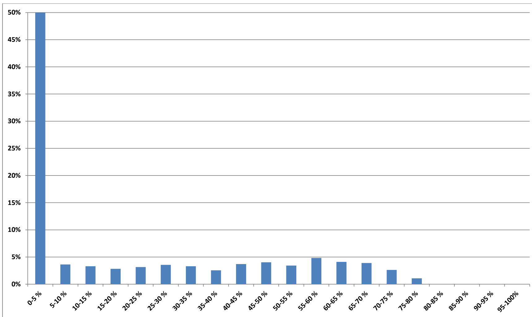
Fig.9 Bretagne Août 2013. Pourcentage du temps en fonction de la puissance solaire livrée (abscisses : intervalles de puissance mesurés en pourcentage de la puissance installée : 142,2 MW). Cette distribution présente la forme « conventionnelle » pour la production solaire d'une zone géographique de petite dimension au regard des zones météo (pas ou peu de foisonnement). L'efficacité moyenne est de 21 % (mois précédent 21,6 %) avec une production qui le 20 du mois à 14h00 a atteint son maximum mensuel d'efficacité 78,2 % (mois précédent 80,1 %). La puissance livrée n'a dépassé 50 % de la puissance moyenne installée que pendant 20 % (mois précédent 19,9 %) du temps. Elle a été inférieure à 15 % de la puissance installée pendant 56,9 % du temps.
