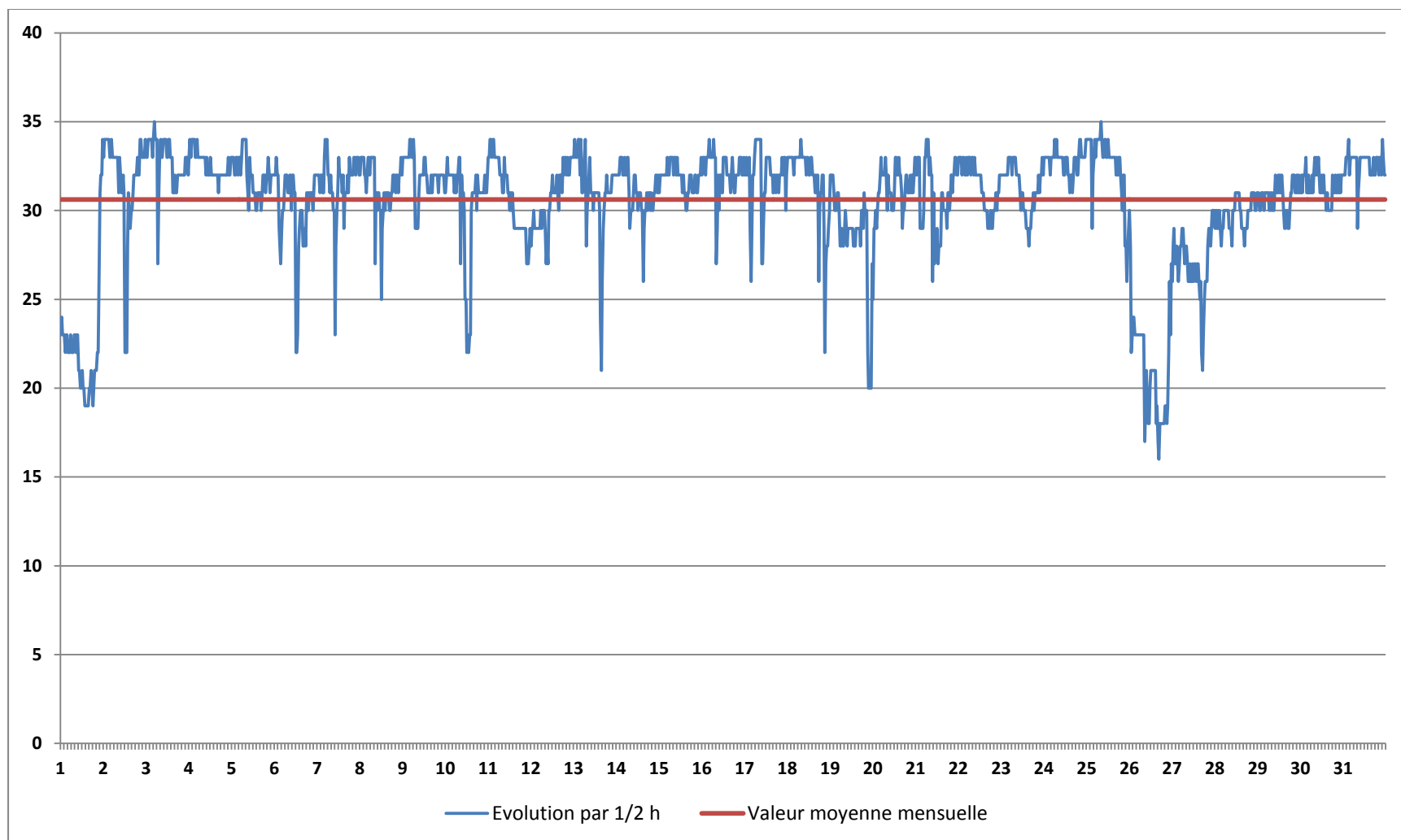
Fig.15 Production ENR thermique, Puissance (MW) Bretagne – Août 2013. Cette production ayant pour origine la combustion de la biomasse et de déchets en cogénération fonctionne comme une énergie de base quasi-constante autour de sa valeur moyenne (30,6 MW). Sur ce mois, le taux de couverture moyen correspondant est de 1,6 % (mois précédent 1,4 %) (variant de 0,7 % à 2,7 %). Une contribution aussi faible ne peut bien sûr pas être utilisée pour la stabilisation du réseau.
