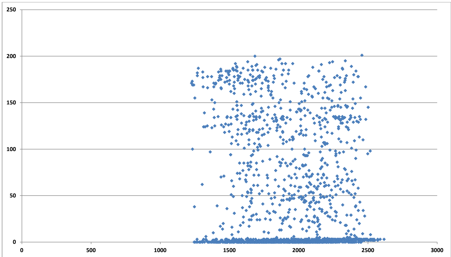
Fig.14 Bretagne Août 2013. Diagramme de corrélation entre la puissance hydraulique livrée (axe vertical unité MW) et la consommation au même instant (axe horizontal MW). Compte tenu de ce que sur une période de l'ordre du mois, il ne peut pas y avoir de corrélation entre les marées avec les besoins électriques de la société on n'observe encore aucune corrélation. L'hydraulique des marées est bien une énergie fatale.
