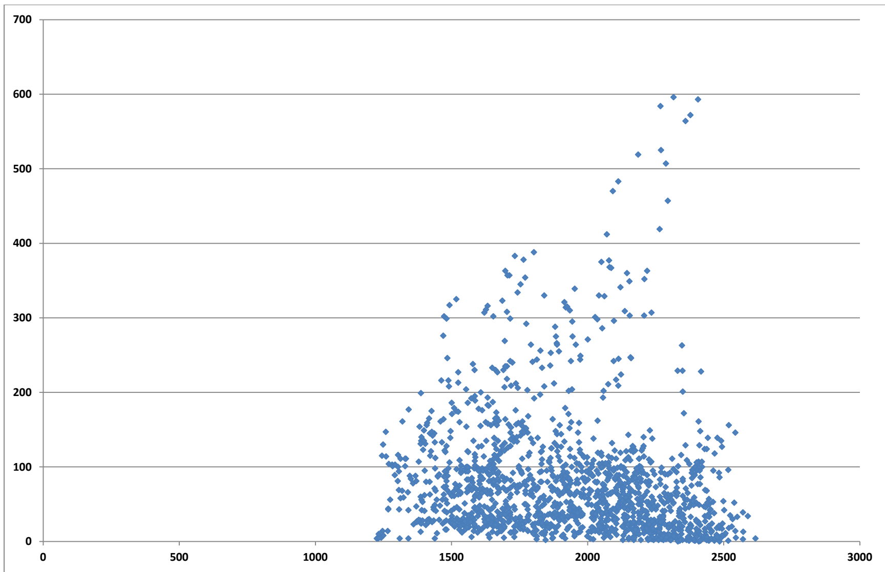
Fig.6 Bretagne Août 2013. Diagramme de corrélation entre la puissance éolienne livrée (axe vertical unité MW) et la consommation au même instant (axe horizontal MW). On n'observe aucune corrélation, comme on pouvait s'y attendre pour une énergie fatale.
