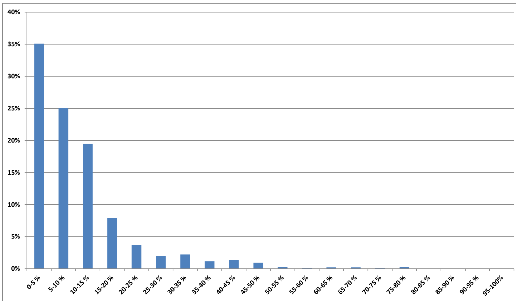
Fig.5 Bretagne Août 2013. Pourcentage du temps en fonction de la puissance éolienne livrée (abscisses : intervalles de puissance mesurés en pourcentage de la puissance installée : 756 MW). Cette distribution décroissante est caractéristique d'une zone géographique de petite dimension au regard des zones météo comme la Bretagne (pas ou peu de foisonnement). Le mois a été exceptionnellement peu productif (efficacité moyenne 10,7 % - mois précédent 15,5 %) avec quelques pics de bonne production au long du mois (quand l'efficacité a atteint 78,8 %). La puissance livrée n'a dépassé 50 % de la puissance moyenne installée que pendant 1,1 % (mois précédent 2,2 %) du temps. Elle a été inférieure à 15 % de la puissance installée pendant 79,6 % (mois précédent 55,4 %) du temps.
