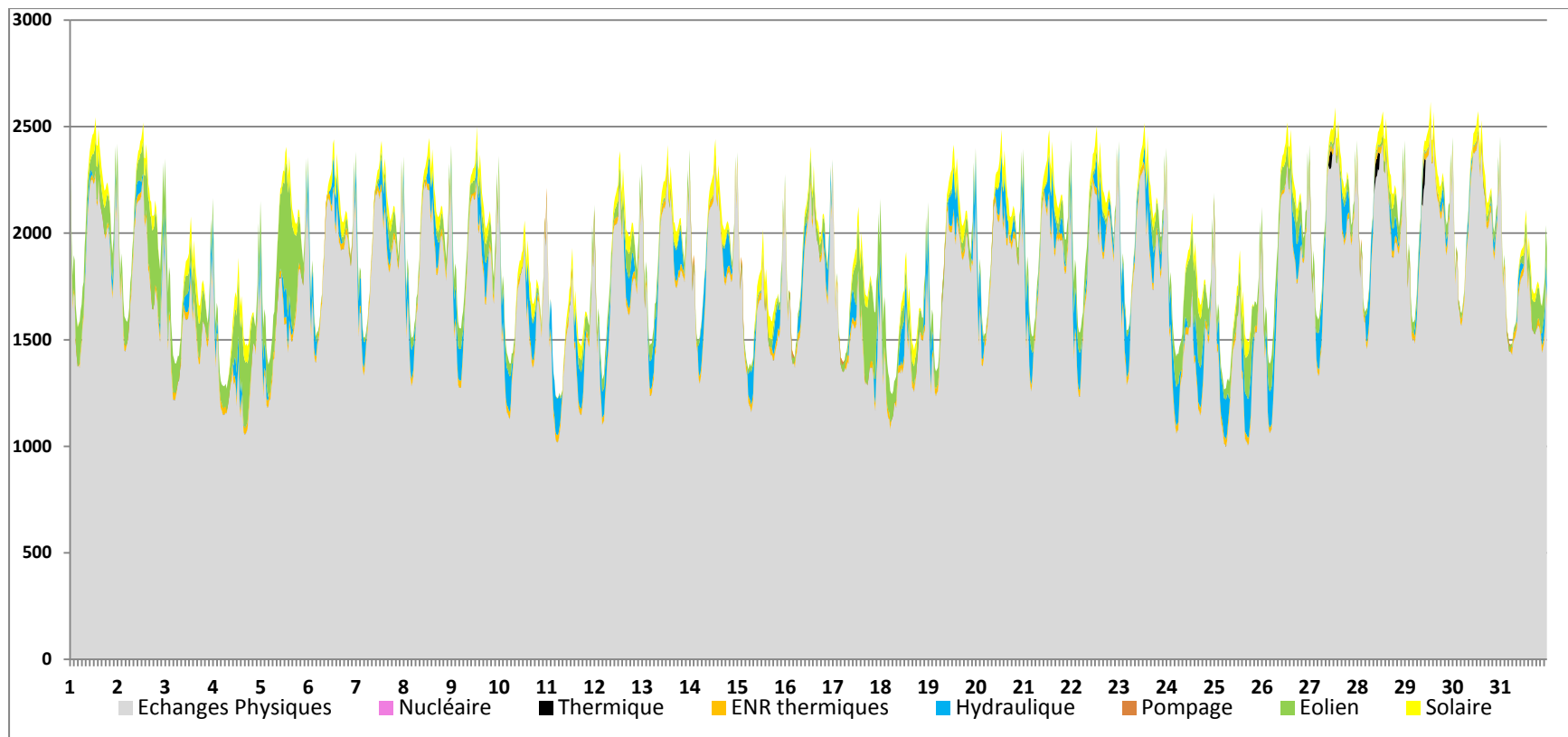
Fig.1 Consommation – production Bretagne Août 2013 (MW). La puissance consommée moyenne du mois a été de 1,93 GW (mois précédent 2,04 GW) entre un maximum de 2,6 GW (mois précédent 2,7 GW) le 29 du mois à 13h00 et un minimum de 1,23 GW (mois précédent 1,25 GW) le 11 du mois à 5h30. La consommation est couverte à 89,9 % (mois précédent 89 %) par des importations. Le complément de production est fourni par l'hydraulique au rythme des marées, par le solaire pour les milieux de journées et par l'éolien, particulièrement sur la première moitié du mois. Les importations oscillent entre 1 et 2,3 GW. La centrale de Flamanville fonctionne à sa puissance nominale (2,5 GW) La capacité d'exportation de la Basse-Normandie est de l'ordre de 1,5 GW – sauf pour les journées 11, 30 et 31 où elle chute à 1 GW. La région Pays-de-Loire a elle importé sans cesse du courant. Les données eCO2mix ne fournissant que le bilan des échanges global sur l'ensemble des frontières régionales permettent difficilement de savoir si de l'énergie électrique produite par les centrales nucléaires en amont sur la Loire, voire des centrales plus lointaines ou de l'étranger, n'a pas traversé cette région – ou la Basse-Normandie – vers la Bretagne. Cela a encore été le cas ce mois-ci.
