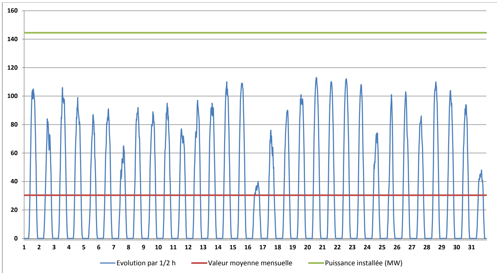
Fig.8 Production photovoltaïque, Puissance (MW) Bretagne – Août 2013. En nous basant sur les données des 30/06/2012 et 30/09/2013 des « Tableaux de bord éolien et photovoltaïque » du ministère nous avons estimé la puissance solaire régionale installée à 144,5 MW. La puissance moyenne livrée au réseau sur le mois a été de 30,4 MW (mois précédent 30,9 MW) soit une efficacité moyenne de 21 % (mois précédent 21,6 %). Le maximum de production a été de 113 MW (mois précédent 115 MW) pour une efficacité 78,2 % (mois précédent 80,1 %) le 20 du mois à 14h00. Les hauteurs des maxima reflètent la variabilité de la nébulosité surimposée à l'évolution astronomique de la hauteur solaire à son zénith. Cette dernière affecte aussi la largeur des pics de production à leur base (maximale au solstice d'été, minimale à celui d'hiver).
