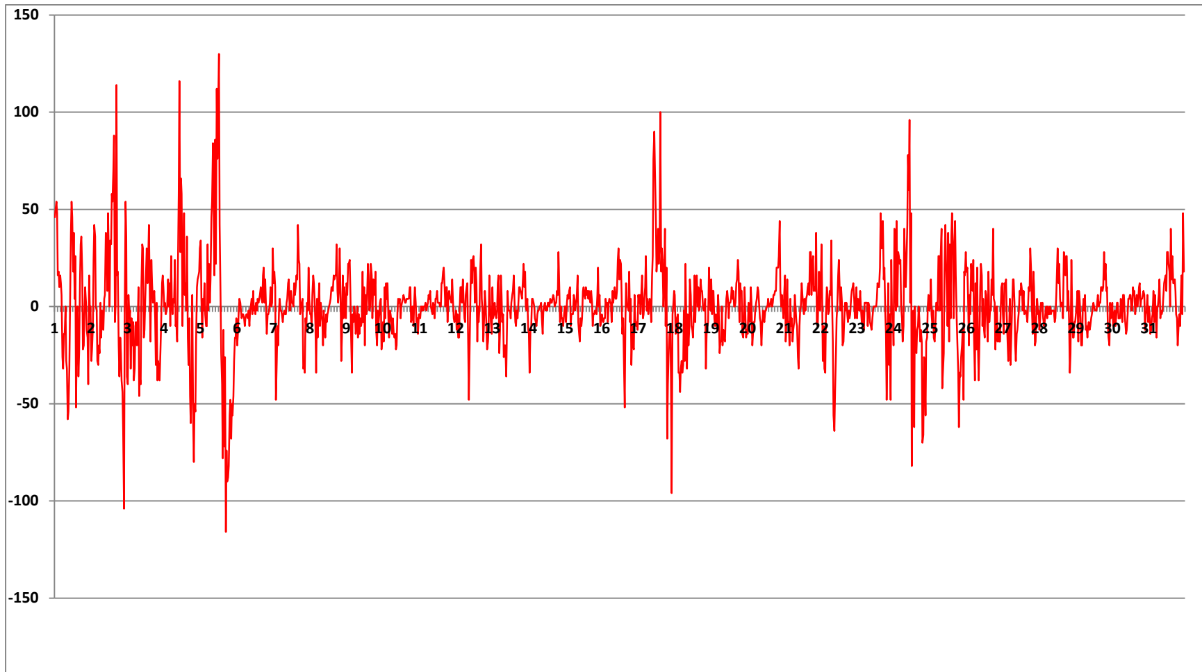
Fig.7 Gradient de puissance éolienne (MW/h) Bretagne – Août 2013. En ce mois très peu venté, le réseau (en fait l'importation de puissance) a dû gérer des gradients de puissance de plus de 100 MW/h aussi bien en positif qu'en négatif.
