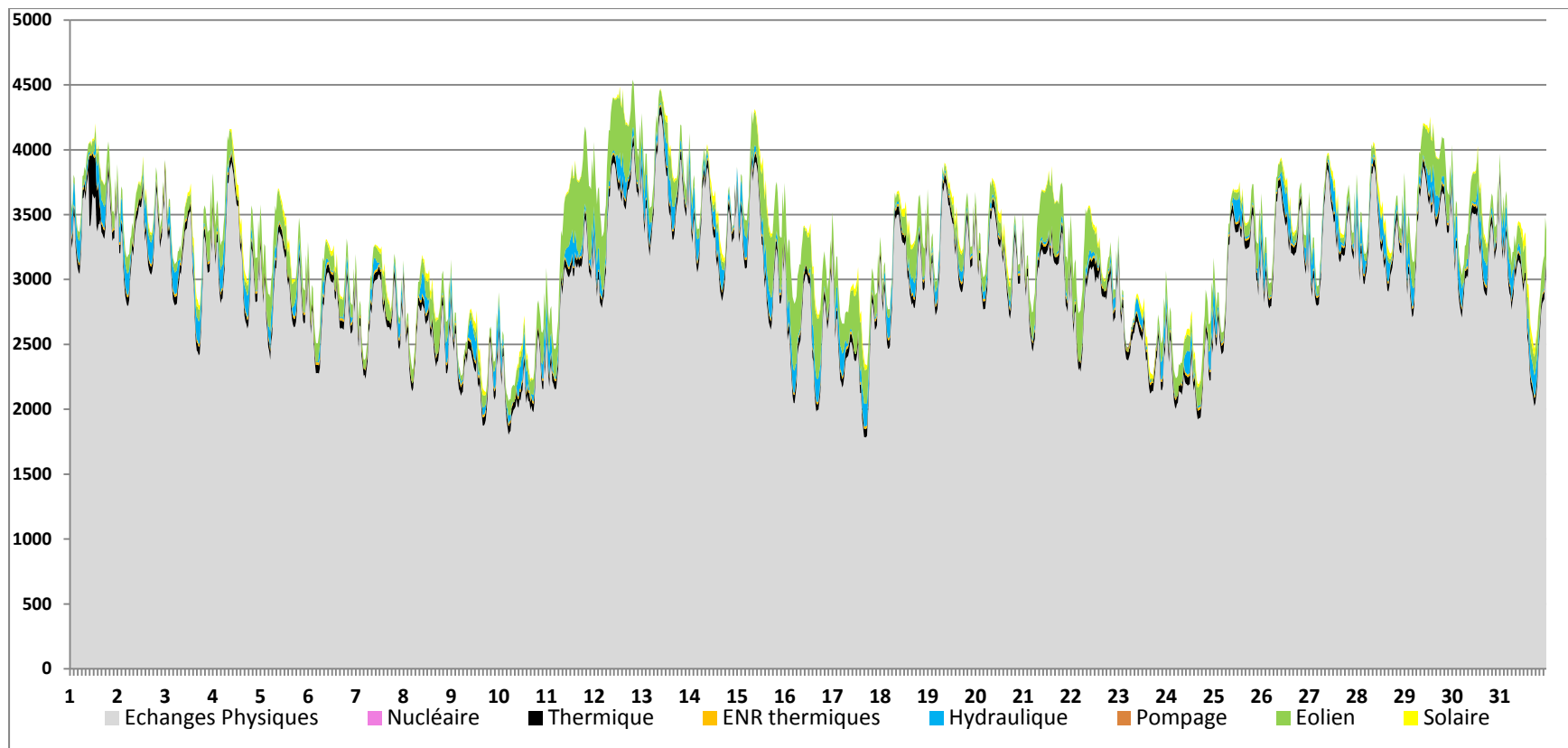
Fig.1 Consommation – production Bretagne Mars 2013 (MW). La puissance consommée moyenne du mois a été de 3,3 GW (mois précédent 3,45 GW) entre un maximum de 4,5 GW (mois précédent 4,3 GW) le 12 du mois à 19h30 et un minimum de 2,1 (mois précédent 2,3 GW) le 10 du mois à 5h00. La consommation est couverte à 90,2 % (mois précédent 90 %) par des importations. Le complément de production est fourni par l'hydraulique au rythme des marées, par le solaire pour les milieux de journées et par l'éolien, particulièrement sur la première moitié du mois. Comme seul un des deux réacteurs de Flamanville (pour 1,3 GW) était en opération, la Basse-Normandie a été importatrice la plupart du temps. La région Pays-de-Loire a elle aussi importé sans cesse du courant. Toutefois, les données eCO2mix ne fournissant que le bilan des échanges global sur l'ensemble des frontières régionales permettent difficilement de savoir si de l'énergie électrique produite par les centrales nucléaires en amont sur la Loire, voire des centrales plus lointaines ou de l'étranger, n'a pas traversé cette région – ou la Basse-Normandie – vers la Bretagne. On a néanmoins la certitude que c'est le cas sur l'ensemble de ce mois.
