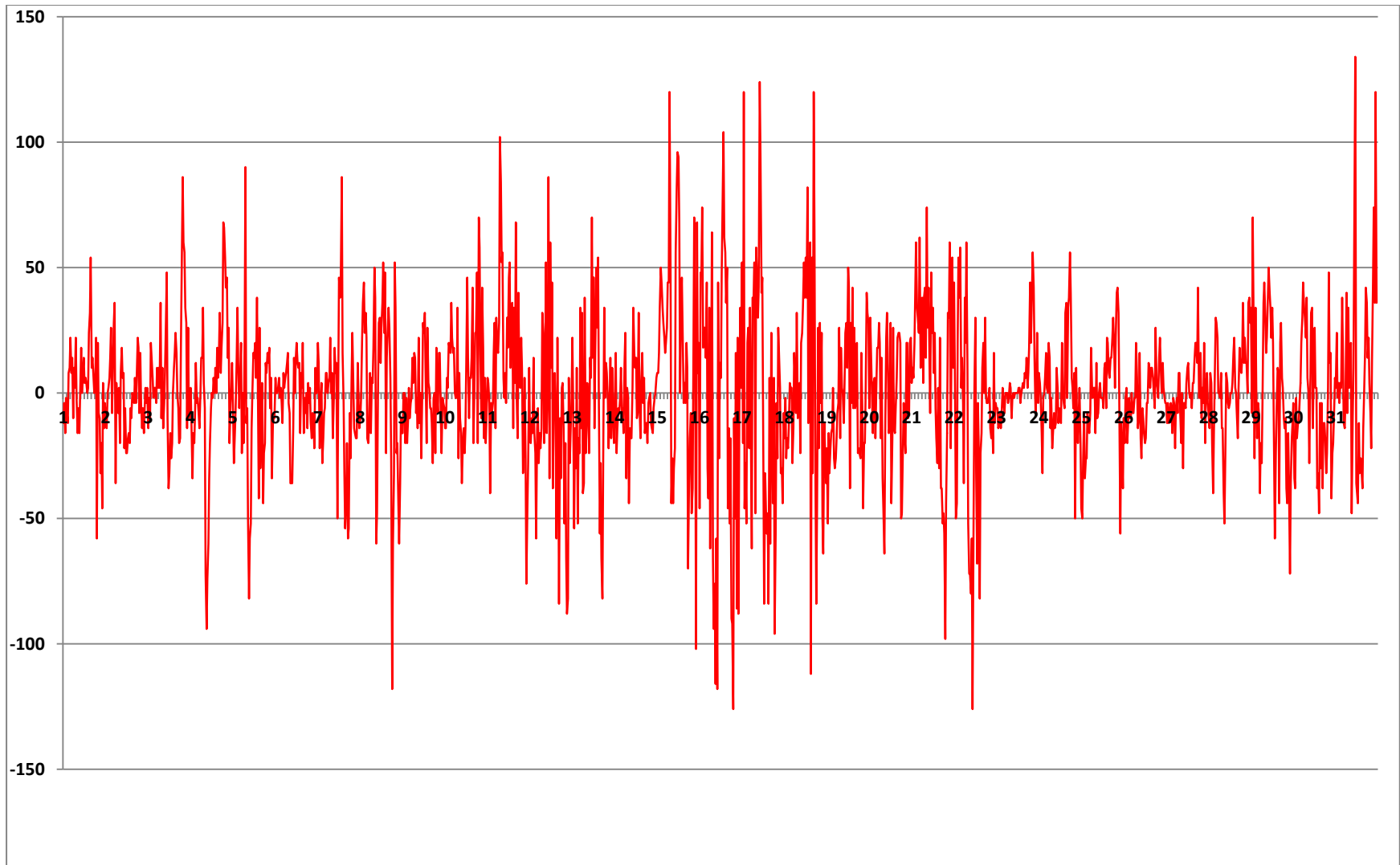
Fig.7 Gradient de puissance éolienne (MW/h) Bretagne – Mars 2013. En ce mois venté surtout dans sa période médiane, la forte production sur la période n'a pas été régulière, Le réseau (en fait l'importation de puissance) a dû gérer des gradients de puissance approchant 130 MW/h aussi bien en positif qu'en négatif.
