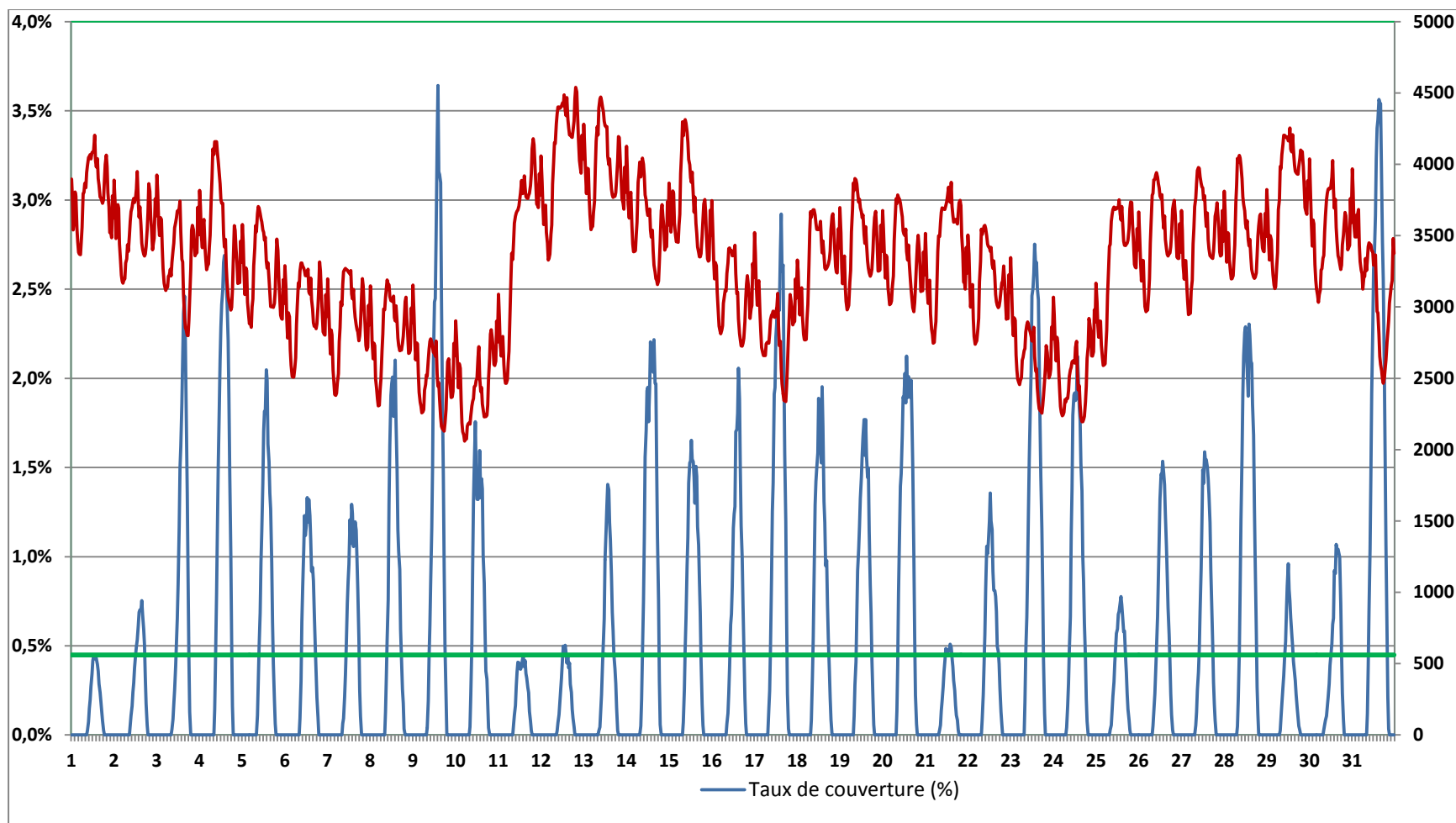
Fig.10 Production photovoltaïque, Taux de couverture (%) Bretagne – Mars 2013. La courbe rouge (échelle de droite en MW) montre l'évolution de la consommation. En moyenne, le taux de couverture (rapport de la puissance livrée à la puissance consommée au même instant) du photovoltaïque est de 0,45 % (mois précédent 0,3 %). Il atteint son maximum de 3,6 % (mois précédent 3,4 %) le 9 du mois à 14h quand le soleil est encore haut et que la consommation baisse. De façon générale, les meilleurs taux de couverture sont atteints les weekends à des moments où une bonne production photovoltaïque se combine à un faible besoin en électricité. Les pics du taux de couverture reflètent donc autant la production solaire que la faible consommation.
