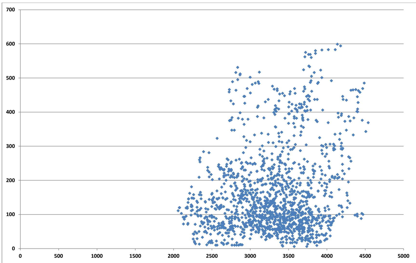
Fig.6 Bretagne Mars 2013. Diagramme de corrélation entre la puissance éolienne livrée (axe vertical unité MW) et la consommation au même instant (axe horizontal MW). On n'observe aucune corrélation, comme on pouvait s'y attendre pour une énergie fatale.
