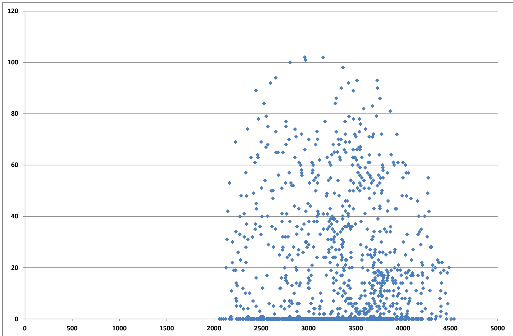
Fig.11 Bretagne Mars 2013. Diagramme de corrélation entre la puissance photovoltaïque livrée (axe vertical unité MW) et la consommation au même instant (axe horizontal MW). On n'observe aucune corrélation, comme on pouvait s'y attendre pour une énergie fatale.
