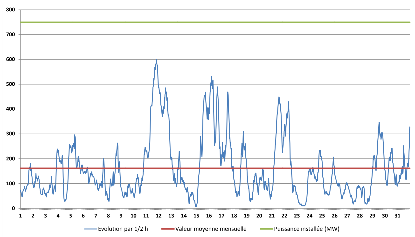
Fig.3 Production éolienne, Puissance (MW) Bretagne – Mars 2013. En nous basant sur les données des 31/12/2012 et 31/03/2013 des « Tableaux de bord éolien et photovoltaïque » du ministère nous avons estimé la puissance éolienne régionale installée à 749,7 MW. La puissance moyenne livrée au réseau sur le mois a été de 161,5 MW (mois précédent 182,9) soit une efficacité moyenne de 21,6 % (mois précédent 24,4 %). Le maximum de production a été de 599 MW (mois précédent 602 MW) pour une efficacité 79,9 % (mois précédent 80,4 %) le 11 du mois à 20h00. Plusieurs fois dans le mois, la production a été quasi-nulle. Elle est descendue à 6 MW le 14 du mois à 23h00.
