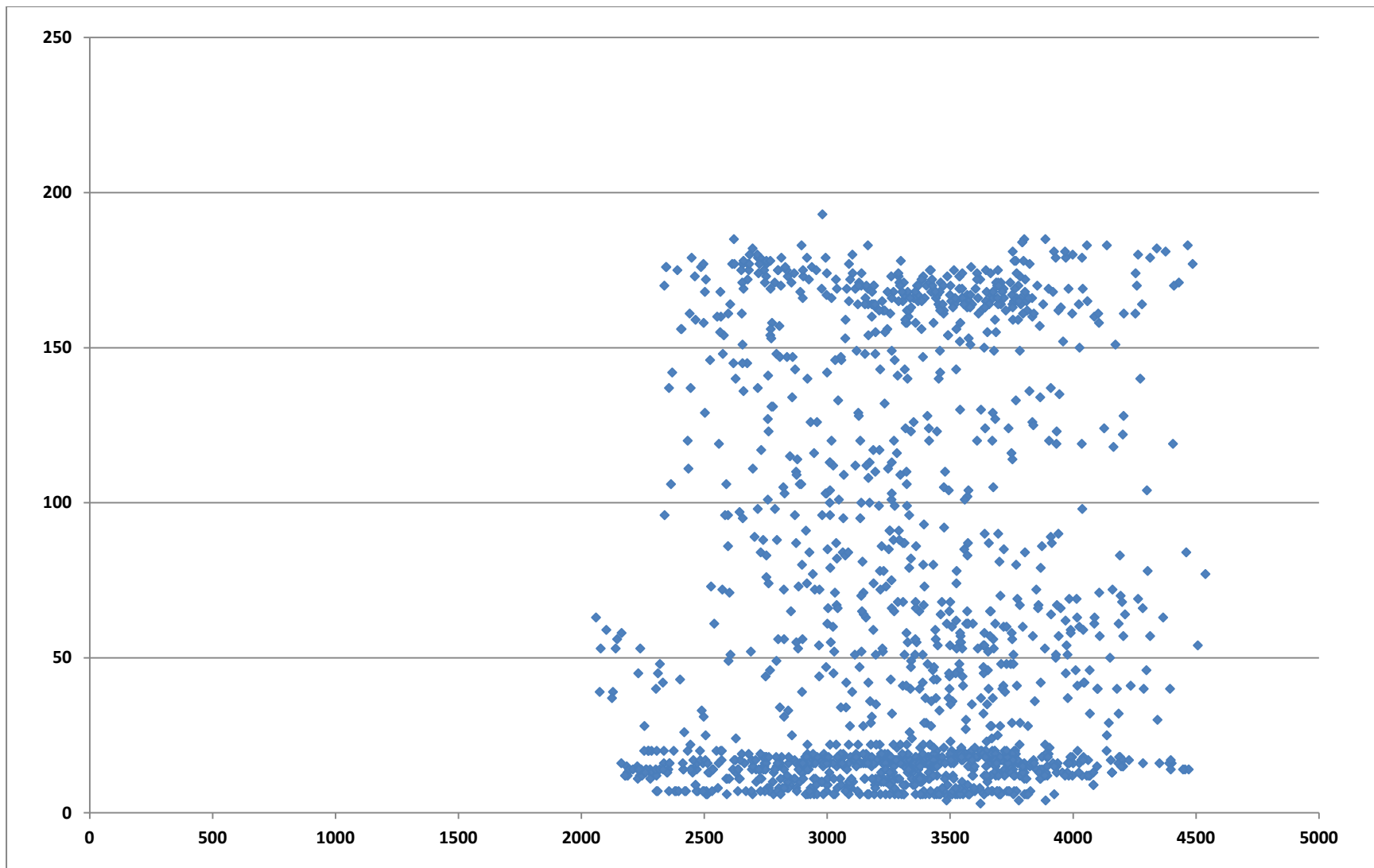
Fig.14 Bretagne Mars 2013. Diagramme de corrélation entre la puissance hydraulique livrée (axe vertical unité MW) et la consommation au même instant (axe horizontal MW). Compte tenu de ce que sur une période de l'ordre du mois, il ne peut pas y avoir de corrélation entre les marées avec les besoins électriques de la société on n'observe encore aucune corrélation. L'hydraulique des marées est bien une énergie fatale.
