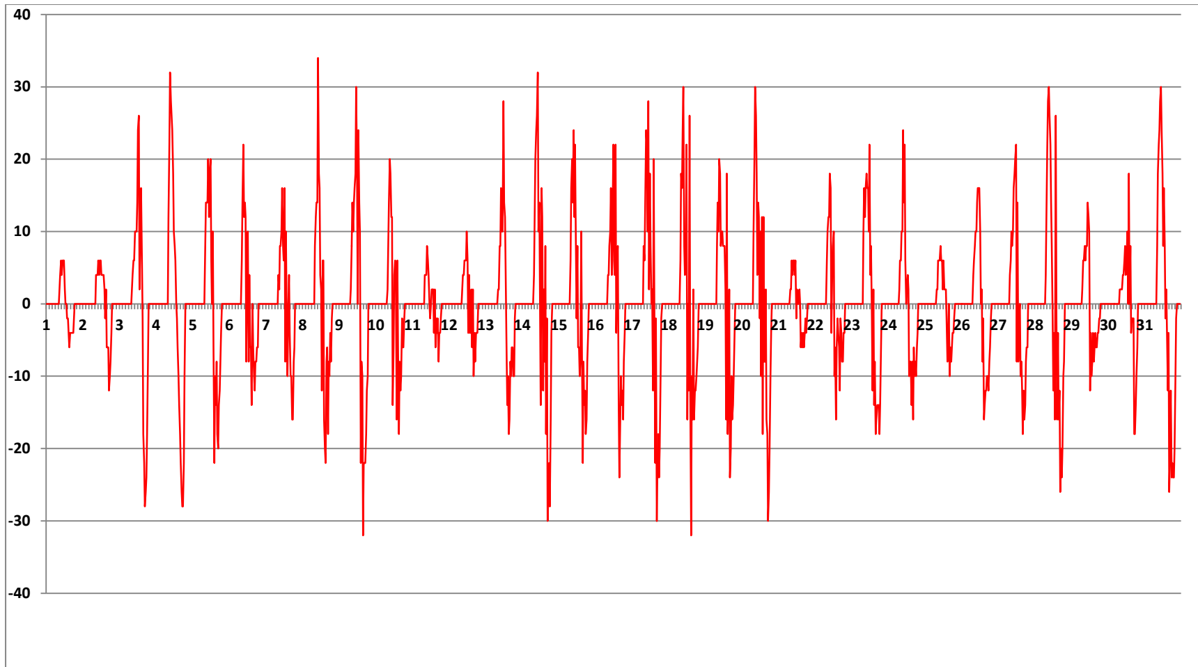
Fig.12 Gradient de puissance solaire (MW/h) Bretagne – Mars 2013 Comme il se doit les gradients sont en moyenne directement liés au pic de production solaire. Ils sont positifs le matin et négatifs l'après-midi. Leur amplitude est aussi en relation avec la hauteur du pic. Plus il y a de soleil, plus le parc photovoltaïque exerce de contrainte sur le réseau. Ainsi pour des pics de moins de 100 MW en milieu de journée les gradients peuvent dépasser +/- 30MW/h. Surimposé à cette tendance générale, on observe aussi des irrégularités à l'échelle de la demi-heure qui, si elles ne correspondent pas une incertitude de la collecte de données par RTE/eCO2mix, pourraient être attribuées à l'effet « un nuage passe ».
