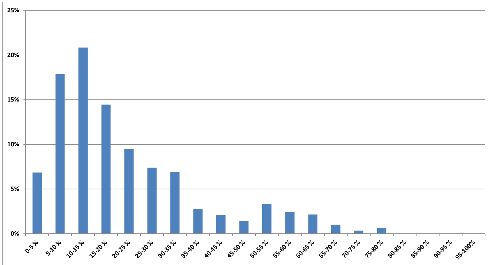
Fig.5 Bretagne Mars 2013. Pourcentage du temps en fonction de la puissance éolienne livrée (abscisses : intervalles de puissance mesurés en pourcentage de la puissance installée : 749,7 MW). Cette distribution en cloche semble indiquer que même sur une zone géographique de petite dimension au regard des zones météo comme la Bretagne il y a eu ce mois-ci un certain effet de foisonnement. Le mois a été moyennement productif (efficacité moyenne 21,6 % - mois précédent 24,4 %) avec un forte période de production (en milieu de mois quand l'efficacité a atteint 79,9 %). La puissance livrée n'a dépassé 50 % de la puissance moyenne installée que pendant 9,95 % (mois précédent 10,1 %) du temps. Elle a été inférieure à 15 % de la puissance installée pendant 45,6 % (mois précédent 38,6 %) du temps.
