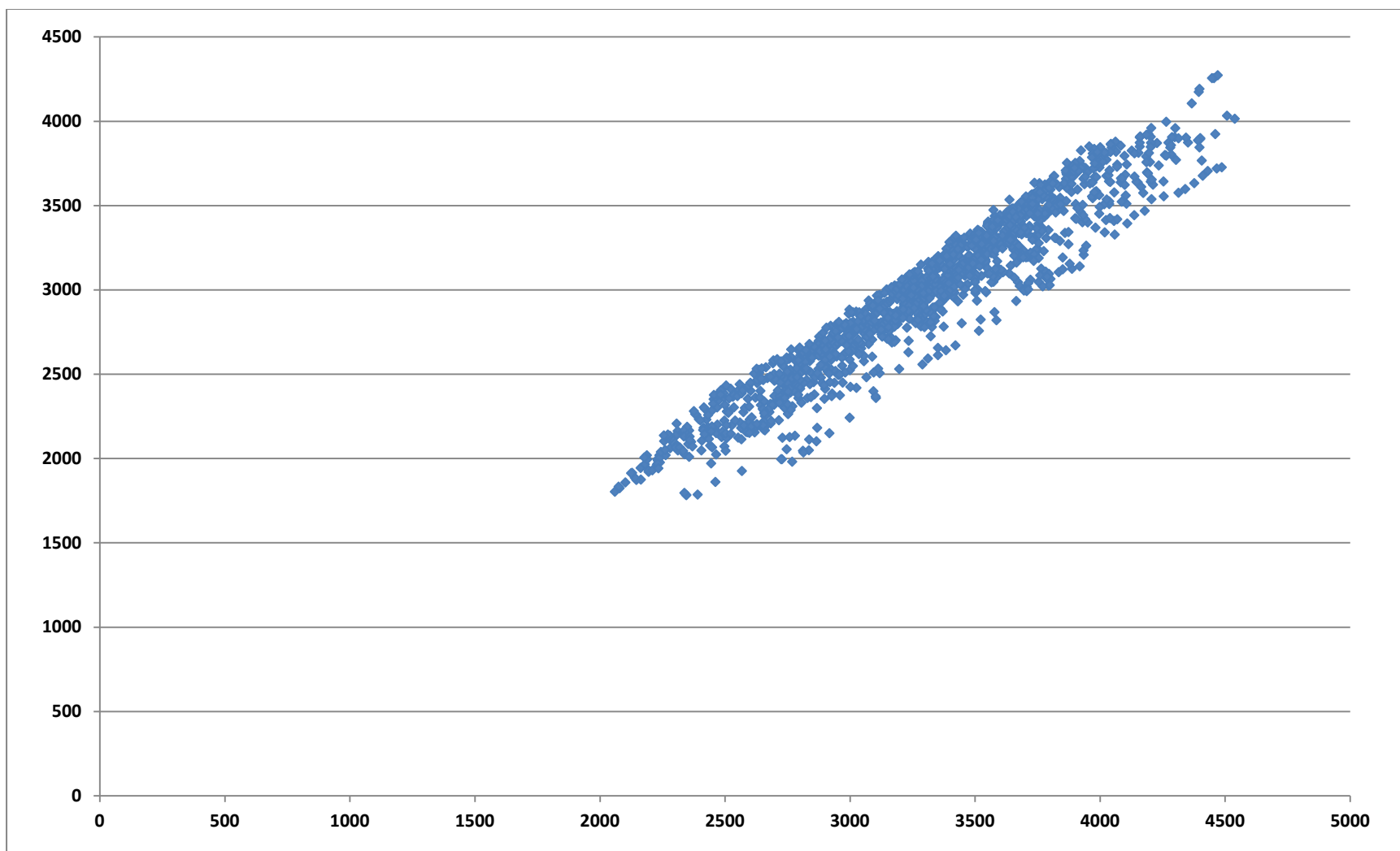
Fig.17 Bretagne Mars 2013. Diagramme de corrélation entre la puissance importée (axe vertical unité MW) et la consommation au même instant (axe horizontal MW). Compte tenu de la dépendance de la région à 90 % de la production importée d'au-delà des régions limitrophes, comme on pouvait s'y attendre, la corrélation est quasi-parfaite.
