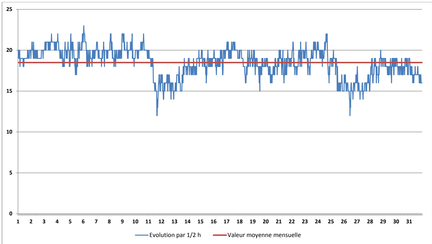
Fig.15 Production ENR thermique, Puissance (MW) Bretagne – Mars 2013. Cette production ayant pour origine la combustion de la biomasse et de déchets en cogénération fonctionne comme une énergie de base quasi-constante autour de sa valeur moyenne (18,5 MW). Sur ce mois, le taux de couverture moyen correspondant est de 0,58 % (mois précédent 0,5 %) (variant de 0,3 % à 1 %). Une contribution aussi faible ne peut bien sûr pas être utilisée pour la stabilisation du réseau.
