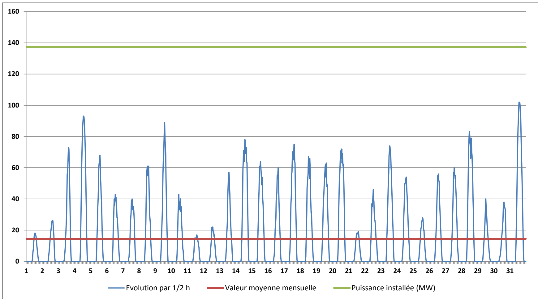
Fig.8 Production photovoltaïque, Puissance (MW) Bretagne – Mars 2013. En nous basant sur les données des 31/12/2012 et 31/03/2013 des « Tableaux de bord éolien et photovoltaïque » du ministère nous avons estimé la puissance solaire régionale installée à 137,2 MW. La puissance moyenne livrée au réseau sur le mois a été de 14,5 MW (mois précédent 11,3 MW) soit une efficacité moyenne de 10,5 % (mois précédent 8,3 %). Le maximum de production a été de 102 MW (mois précédent 95 MW) pour une efficacité 74,34 % (mois précédent 70,1 %) le 31 du mois à 13h30. Les hauteurs des maxima reflètent la variabilité de la nébulosité surimposée à l'évolution astronomique de la hauteur solaire à son zénith. Cette dernière affecte aussi la largeur des pics de production à leur base (maximale au solstice d'été, minimale à celui d'hiver).
