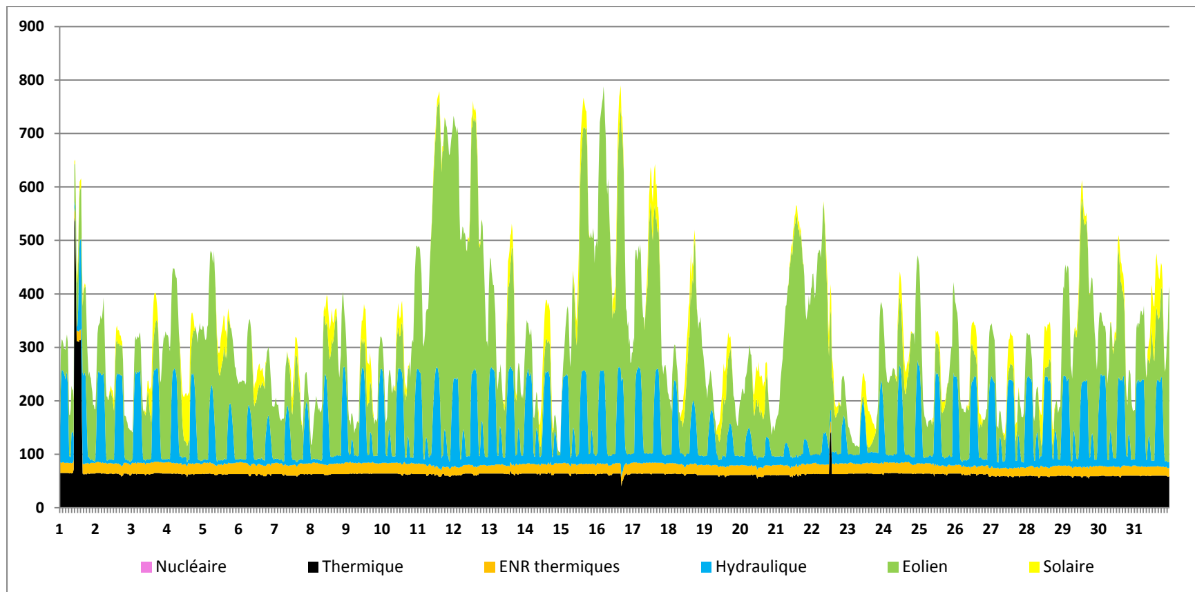
Fig.2 Production électrique de la Bretagne Mars 2013 (MW). Ce mois-ci, l'ensemble de ces productions compte environ 10 % de la consommation locale. En GWh la production totale a été de 120,2 (mois précédent 122,9) pour l'éolien, 50 (mois précédent 47,3) pour l'hydraulique, 13,8 (mois précédent 12,8) pour les ENR thermiques et de 10,8 (mois précédent 7,6) pour le solaire (consommation totale 2457,3 GWh – mois précédent 2319,4 GWh). A l'exception des ENR Thermiques dont la production est quasi-constante et de la faible contribution thermique (48 GWh – mois précédent 43,4 GWh), les autres énergies, toutes fatales, fluctuent sans corrélation avec les besoins en électricité de la région. La production constante de l'énergie thermique s'explique par l'attrait financier de subventions spécifiques accordées à la cogénération en période hivernale (Novembre à Mars). A l'exception de quelques pics (dont l'un atteint, pendant quelques heures, une valeur voisine de 250 MW d'amplitude !) le thermique (comme l'ENR thermique) fonctionne en base sans participer à la gestion de régulation du réseau.
