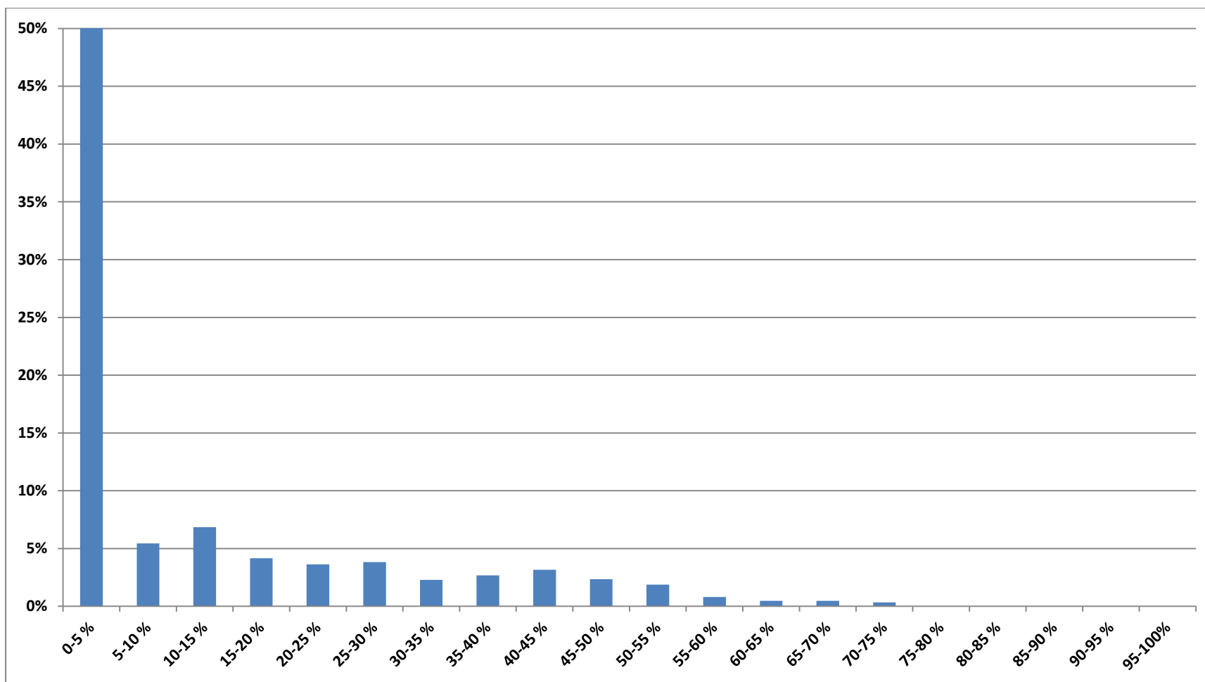
Fig.9 Bretagne Mars 2013. Pourcentage du temps en fonction de la puissance solaire livrée (abscisses : intervalles de puissance mesurés en pourcentage de la puissance installée : 137,2 MW). L'axe vertical a été tronqué à 50 %. La barre la plus à gauche s'élève en fait à 62 %. Cette distribution présente la forme « conventionnelle » pour la production solaire d'une zone géographique de petite dimension au regard des zones météo (pas ou peu de foisonnement). L'efficacité moyenne est de 10,54 % (mois précédent 8,3 %) avec une production qui le 31 du mois à 13h30 a atteint son maximum mensuel d'efficacité 74,3 % (mois précédent 70,1 %). La puissance livrée n'a dépassé 50 % de la puissance moyenne installée que pendant 3,97 % (mois précédent 4,1 %) du temps. Elle a été inférieure à 15 % de la puissance installée pendant 73,9 % du temps.
