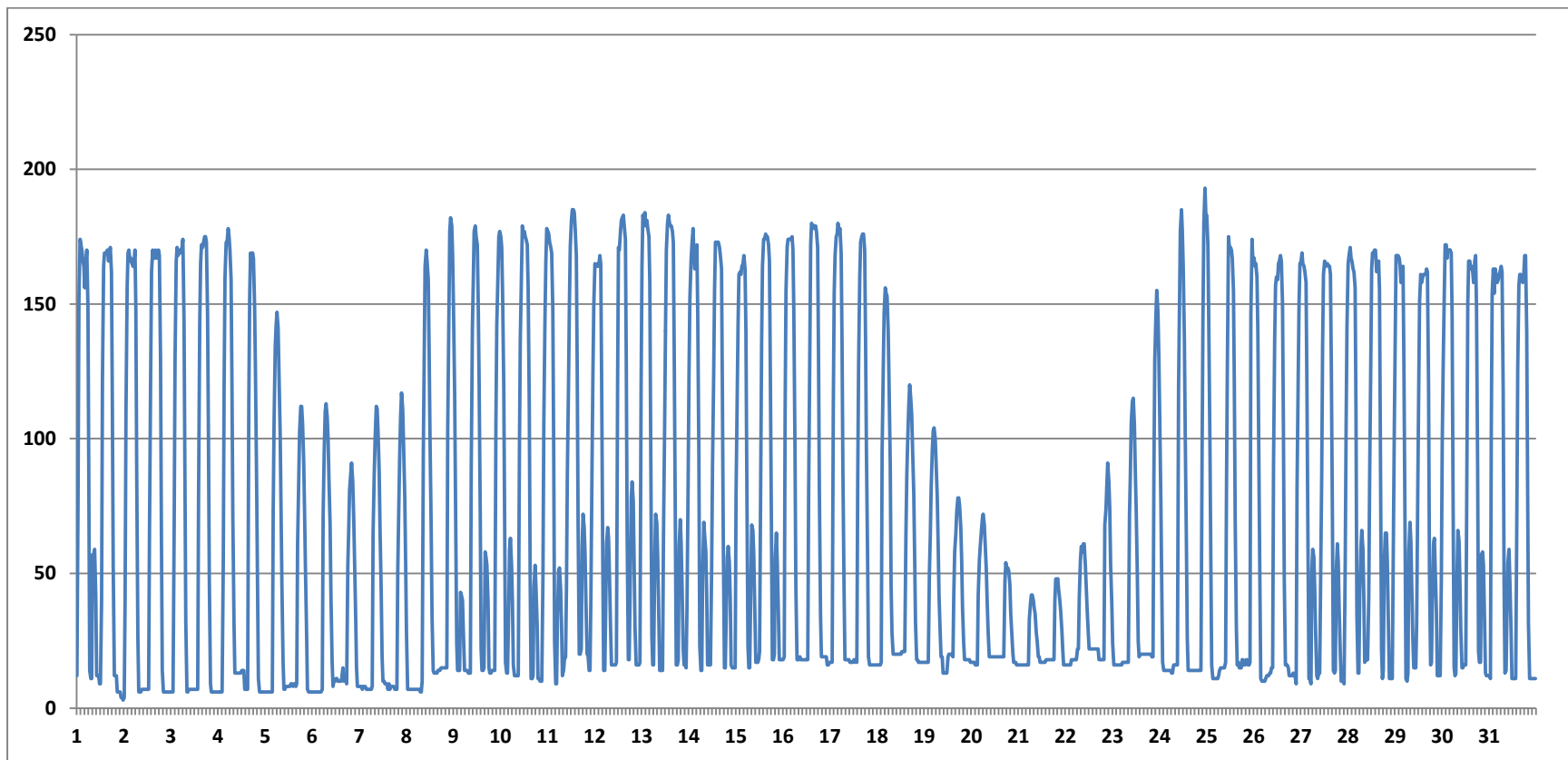
Fig.13 Production hydraulique, Puissance (MW) Bretagne – Mars 2013. L'hydraulique breton lié au barrage de la Rance se distingue du reste de l'hydraulique français (de type « fil de l'eau » ou « éclusées »). C'est non seulement une énergie fatale (comme l'hydraulique de fil de l'eau) mais aussi une production au rythme alternatif. Elle ne participe que faiblement au réglage du réseau par le biais d'une fonction de pompage. L'énergie totale livrée au réseau sur le mois a été de 50 GWh (mois précédent 47,3 GWh), alors que le pompage (une consommation de courant restituée pour partie ultérieurement et comptabilisée dans le total « hydraulique ») n'a concerné que 3,7 GWh. Difficilement visible sur cette figure, on peut vérifier un décalage horaire progressif des pics reflétant celui des marées (idem pour les pics de pompage non illustrés dans ce document). Les structures de production à « pic double » observable en milieu et fin de mois, correspondant à des périodes où il y a peu de stockage par pompage.
