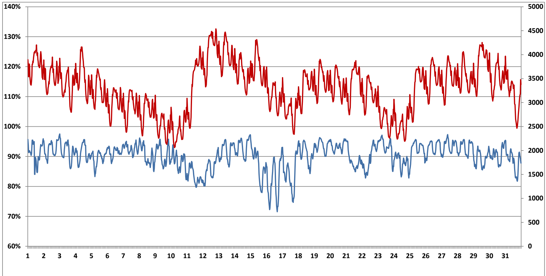
Fig.16 Importation électrique, Taux de couverture (%) Bretagne – Mars 2013. La courbe rouge (échelle de droite en MW) montre l'évolution de la consommation. En moyenne sur le mois, le taux de couverture (rapport de cette puissance importée à la puissance consommée par la région au même instant) est de 90,2 % (mois précédent 90 %). A son maximum il atteint 97,5 % (mois précédent 98,5 %) le 3 du mois à 00h00. Au minimum, le taux de couverture d'importation est de 71,5 % (mois précédent 71,8 %). Il a lieu le 16 du mois à 16h00 au moment où en ce jour de week-end le taux de couverture éolien s'approche de 20 %.
