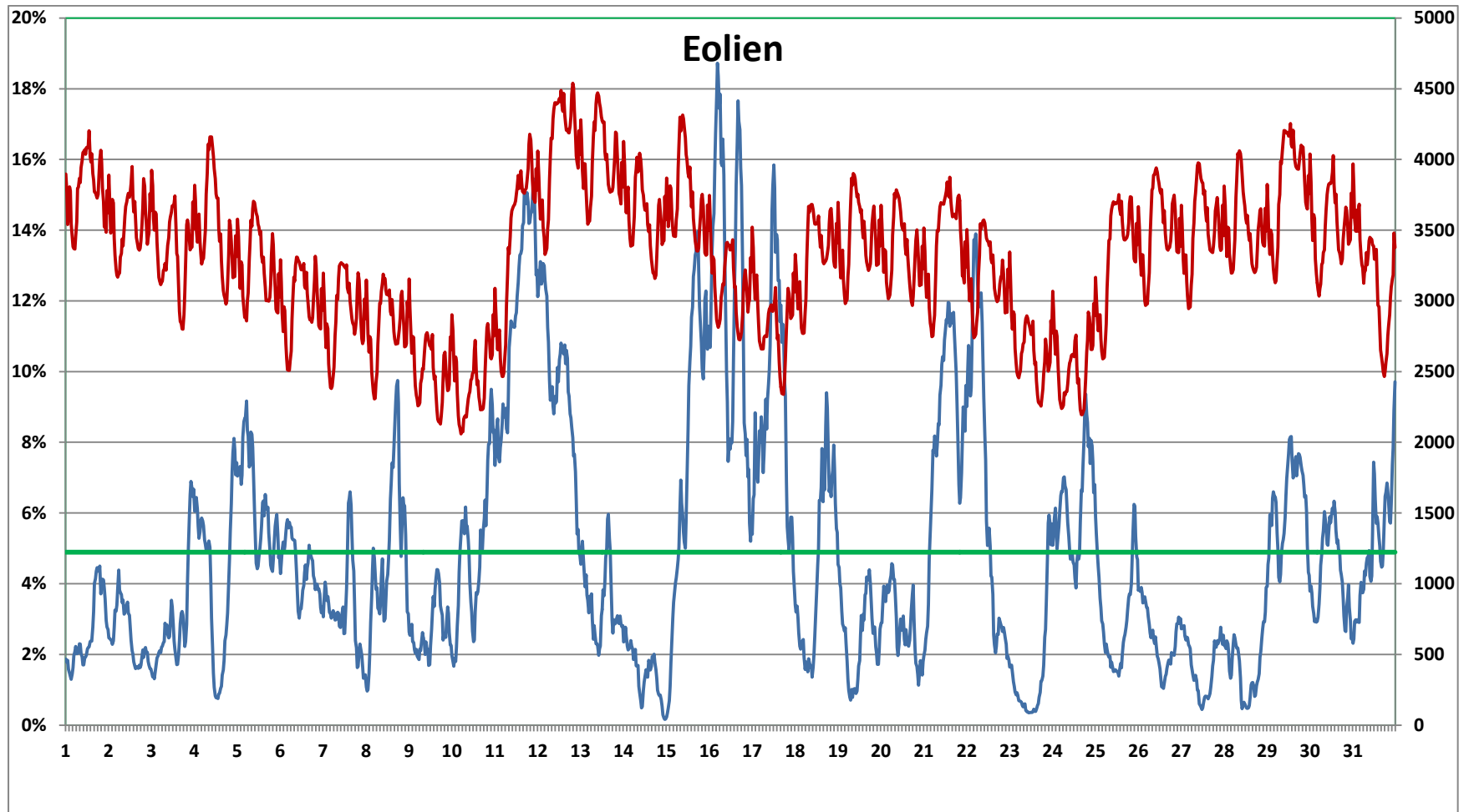
Fig.4 Production éolienne, Taux de couverture (%) Bretagne – Mars 2013. La courbe rouge (échelle de droite en MW) montre l'évolution de la consommation. En moyenne, le taux de couverture (rapport de la puissance livrée à la puissance consommée au même instant) de l'éolien est de 4,9 % (mois précédent 5,4 %). Il atteint son maximum de 18,7 % (mois précédent 20 %) le 16 du mois à 4h30 du matin (une nuit de weekend) à un moment qui combine une forte production éolienne et un faible besoin en électricité. Les pics du taux de couverture reflètent donc autant la production éolienne que la faible consommation. Le minimum est de 0,16 % le 14 du mois à 23h00 (un jour ouvré).
